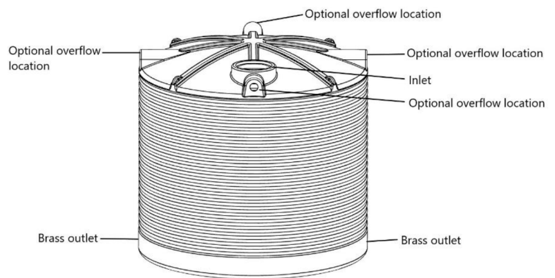
RWT10000
